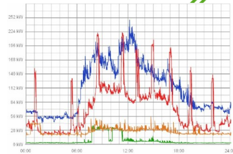
Aufnahme der Lastkurve in Zusammenarbeit mit Electrosuisse
